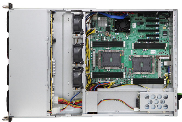
Backplane
